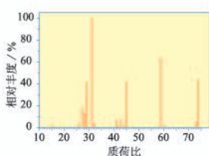
图1 质谱
