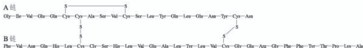
图4-13 牛胰岛素的一级结构示意图（图中使用了氨基酸的缩写，如甘氨酸根据其英文名glycine缩写为Gly）
