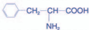
苯丙氨酸（2-氨基-3-苯基丙酸）
