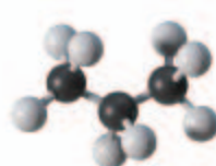
丙烷
