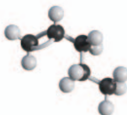
1-戊烯
