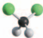
图1-6 二氯甲烷的分子结构模型
