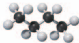
正丁烷
