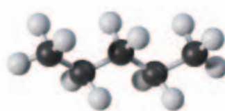
正戊烷
