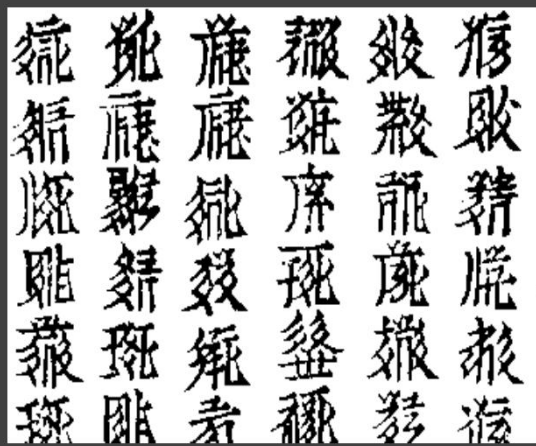
西夏文
