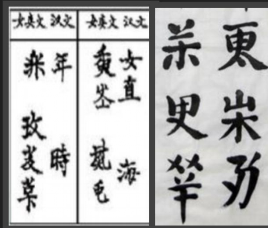
女真文
