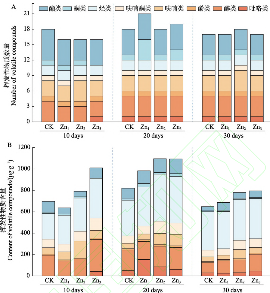
图 3 不同锌肥处理挥发性物质的数量 (A) 和含量比较 (B)
